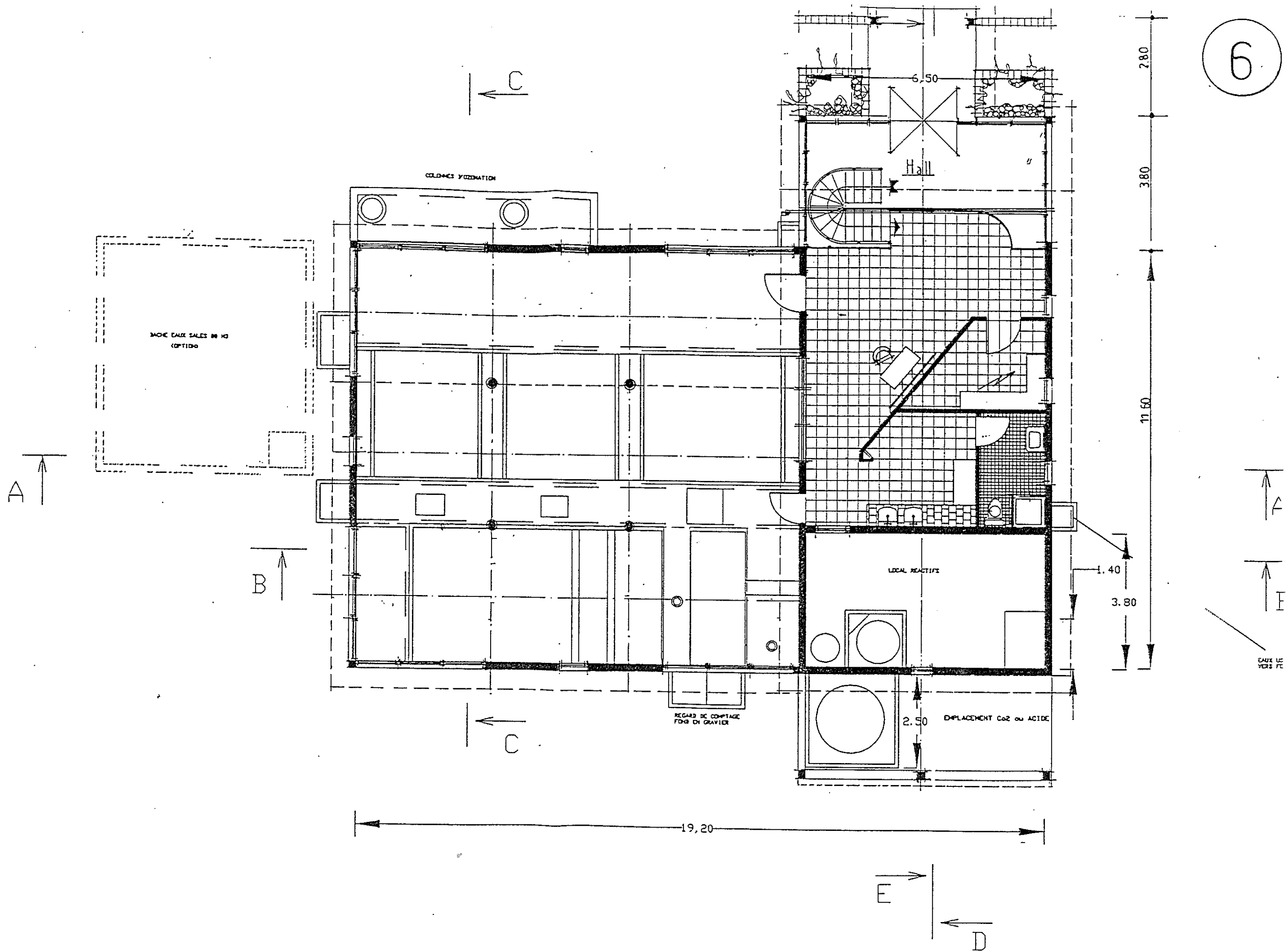
Plan Etage
