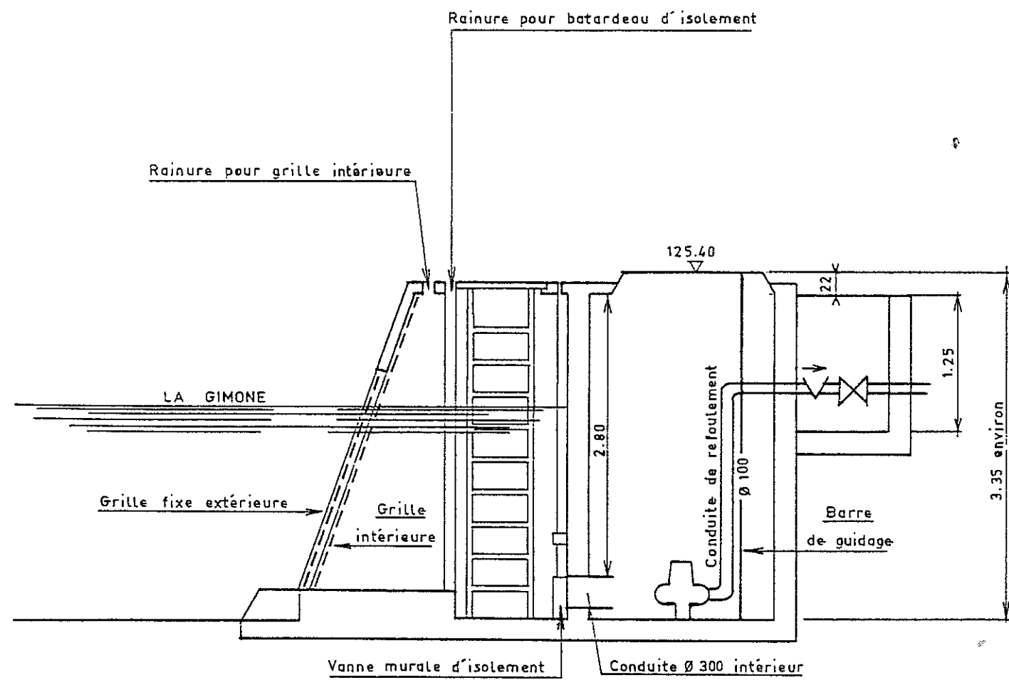
Coupe de la prise d'eau existante
